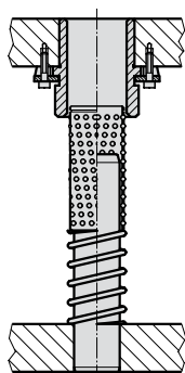
ohne Käfighalter
