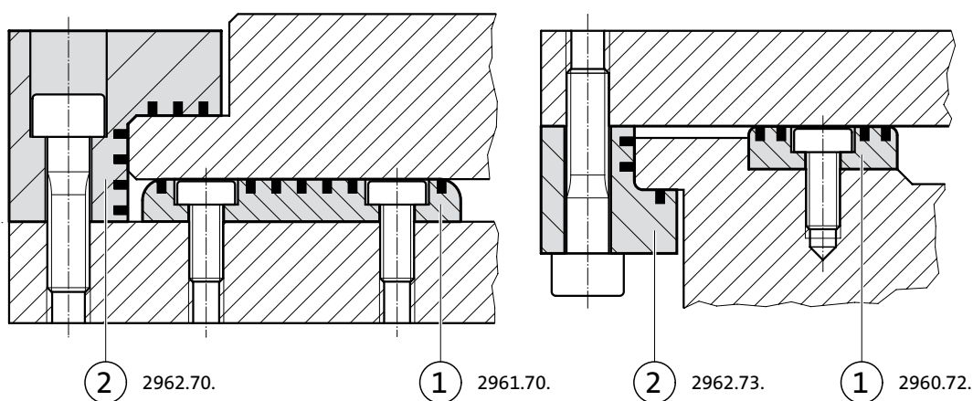
Pos. 1 2961.70. Flachleiste 2960.72. Gleitplatte Mini
