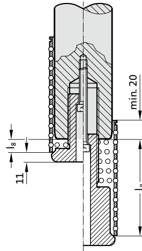
Einbaubeispiel
