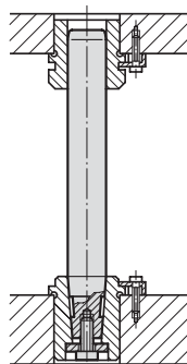
Einbaubeispiel
