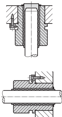
Einbaubeispiel
