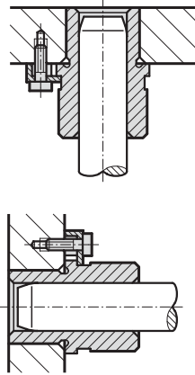
Einbaubeispiel
