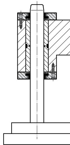
Einbaubeispiel
