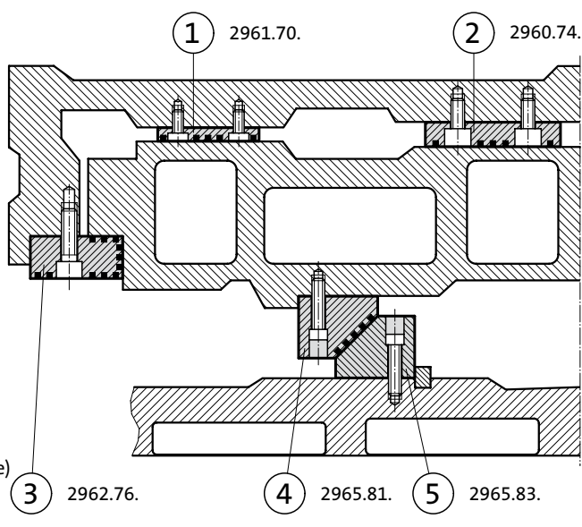
Pos. 3 2962.76. Führungsleiste mit drei Gleitflächen
