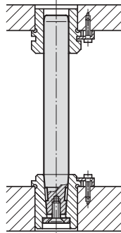
Einbaubeispiel
