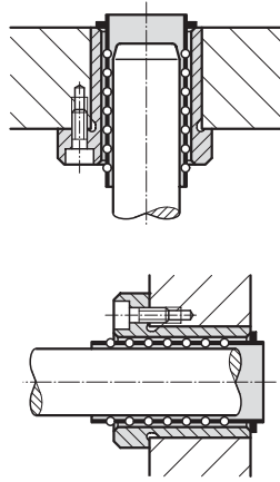
Einbaubeispiel
