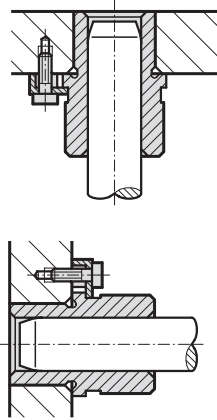
Einbaubeispiel
