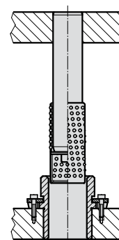
mit Käfighalter 202.92.1.
