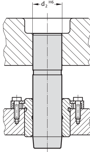
Einbaubeispiel
